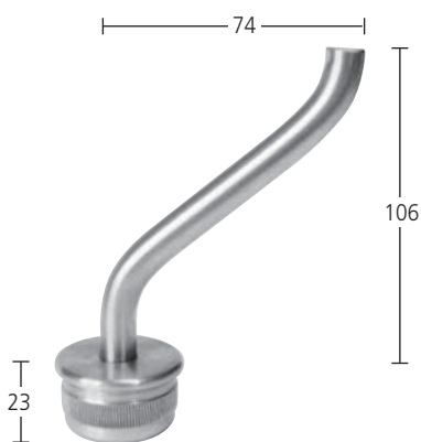
Rohraufsatz für Rohr 42,4 mm Stift 12 mm, Stopfen gerändelt Art. 6.01.0320
