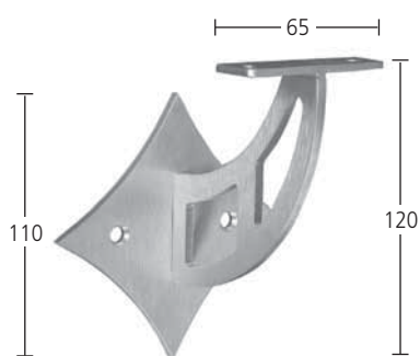
Handlaufträger Materialstärke 4 mm Wandabstand 75 mm mit gewölbter Platte Art. 6.01.8090
