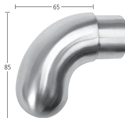
Handlauf-Abschluss V4A für Rohr 42,4 mm Art. 6.01.4390
