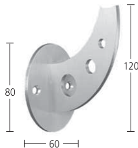
Handlaufträger für Rohr 42,4 mm Materialstärke 4 mm Wandabstand 79 mm Art. 6.01.8040
