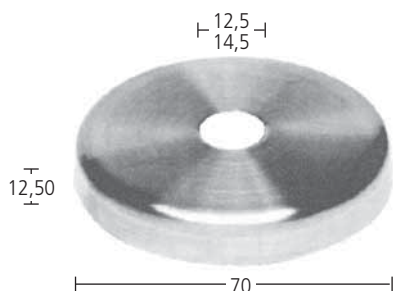
Abdeckrosette Bohrung 12,5 mm Art. 6.01.2000 Bohrung 14,5 mm Art. 6.01.2010
