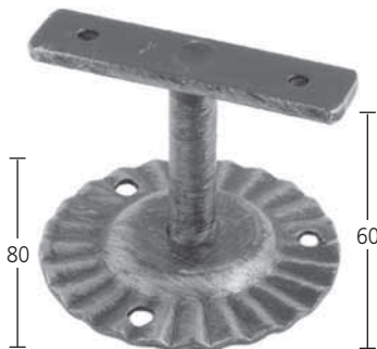
Handlaufträger Art. 4.09.0110
