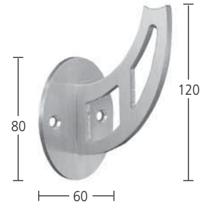
Handlaufträger für Rohr 42,4 mm Materialstärke 4 mm Wandabstand 79 mm Art. 6.01.8050
