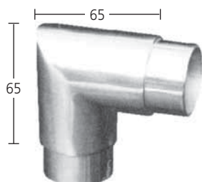
Rohr-Verbinder V4A für Rohr 42,4 / 2 mm Art. 6.01.4250
