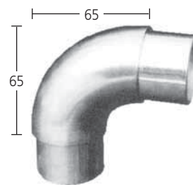
Rohr-Verbinder V4A für Rohr 42,4 / 2 mm Art. 6.01.4200
