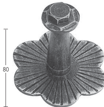
Handlaufträger Wandabstand 80 mm mit Stockschraube M 10 x 160 mm Art. 4.09.0160
