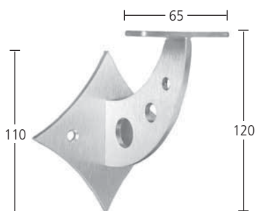
Handlaufträger Materialstärke 4 mm Wandabstand 75 mm mit gerader Platte Art. 6.01.8120
