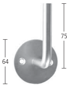
Handlaufträger ohne Gewinde Stift 12 mm, Loch gesenkt Art. 6.01.0060
