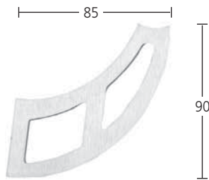
Handlaufträger zum Anschweißen für Rohr 42,4 mm Materialstärke 4 mm Wandabstand 75 mm Art. 6.01.8000
