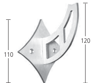
Handlaufträger für Rohr 42,4 mm Materialstärke 4 mm Wandabstand 79 mm Art. 6.01.8020
