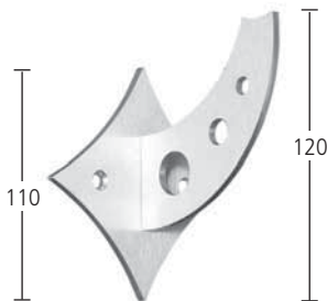
Handlaufträger für Rohr 42,4 mm Materialstärke 4 mm Wandabstand 79 mm Art. 6.01.8030
