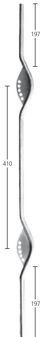
Geländerstab Ø 12 mm Art. 6.05.0300 Ø 14 mm Art. 6.05.0301
