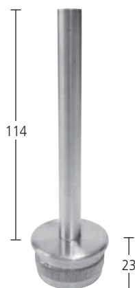
Rohraufsatz Stift 12 mm, Stopfen gerändelt für Rohr 42,4 / 2 mm Art. 6.01.0340
