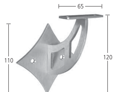
Handlaufträger Materialstärke 4 mm Wandabstand 75 mm mit gerader Platte Art. 6.01.8080
