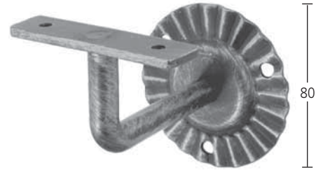
Handlaufträger Wandabstand 80 mm Art. 4.09.0100
