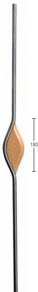
Geländerstab Ø 14 mm Buche lackiert Art. 6.05.0510
