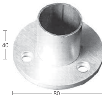
Wand/Bodenanker ohne Klemmschrauben, roh für Rohr 42,4 / 2 mm Art. 6.01.3970
