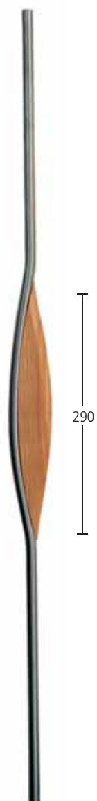
Geländerstab Ø 14 mm Buche lackiert Art. 6.05.0500
