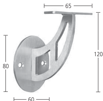
Handlaufträger Materialstärke 4 mm Wandabstand 75 mm mit gerader Platte Art. 6.01.8100
