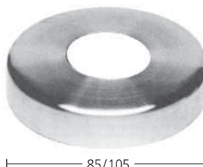
Abdeckrosette Ø 85 mm, Höhe 14 mm, Bohrung 42,4 mm Art. 6.01.2040 Ø 105 mm, Höhe 22,5 mm, Bohrung 42,4 mm Art. 6.01.2050
