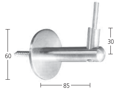
Handlaufträger 3-teilig komplett für Wandmontage mit Stockschraube und Dübel Art. 6.01.0210
