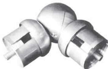
Gelenk-Rohr-Verbinder V2A Rohr zu Rohr 42,4 / 2 mm Kugel verdrehbar, kann an verschiedene Rohrstärken angepasst werden, verstellbar 90–270° Haubenverschluss für Rohre Art. 6.01.4500
