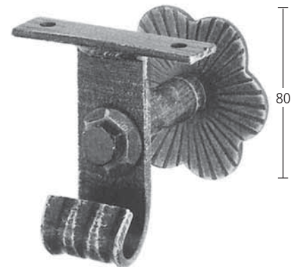
Handlaufträger Wandabstand 65 mm Art. 4.09.0180
