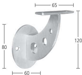
Handlaufträger Materialstärke 4 mm Wandabstand 75 mm mit gerader Platte Art. 6.01.8060
