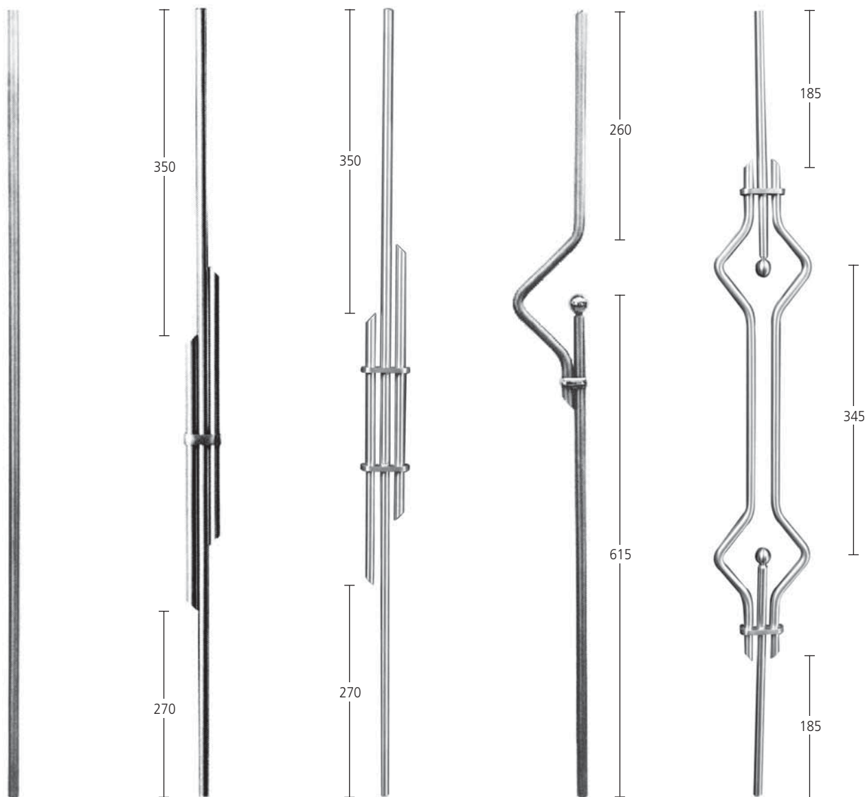
Geländerstab Ø 12 mm Art. 6.05.0020
