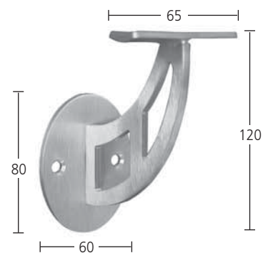
Handlaufträger Materialstärke 4 mm Wandabstand 75 mm mit gewölbter Platte Art. 6.01.8110
