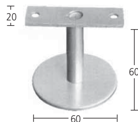
Handlauf-Stütze für Brüstung mit gerader Platte Art. 6.01.0410
