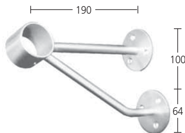
Fuss-Stütze für Rohr 42,4 mm Wandbefestigung Art. 6.01.0310
