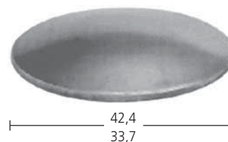
Anschweiss-Kappe roh, Stärke 2 mm, für Rohr 42,4 mm Art. 6.01.1350 für Rohr 33,7 mm Art. 6.01.1360
