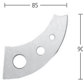
Handlaufträger zum Anschweißen für Rohr 42,4 mm Materialstärke 4 mm Wandabstand 75 mm Art. 6.01.8010
