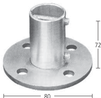
Wand/Bodenanker mit Klemmschrauben, roh für Rohr 42,4 / 2 mm Art. 6.01.3900 für Rohr 33,7 / 2,6 mm Art. 6.01.3930
