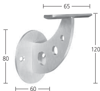
Handlaufträger Materialstärke 4 mm Wandabstand 75 mm mit gewölbter Platte Art. 6.01.8070
