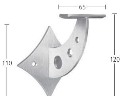
Handlaufträger Materialstärke 4 mm Wandabstand 75 mm mit gewölbter Platte Art. 6.01.8130
