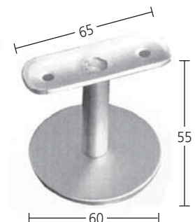
Handlauf-Stütze für Brüstung mit gewölbter Platte Art. 6.01.0420
